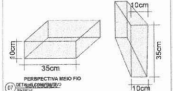
(07) PERSPECTIVA MEIO FIO
