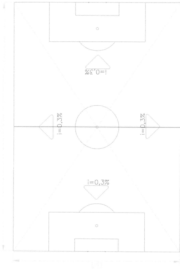
DIAGRAMA DE DREAGEM SUPERFICIAL ESC.: SEM ESCALA
