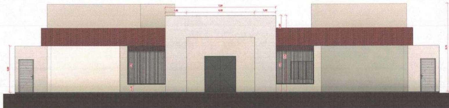
1 Fachada Escala: 1/30
